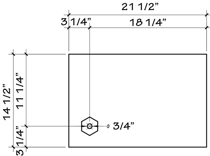
TOP/ VENT
